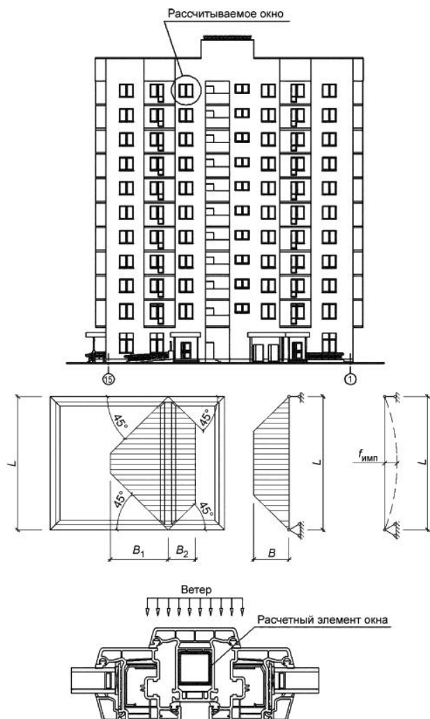
Рисунок Б.4 - Расчетная схема для определения жесткости оконных блоков при действии равномерно распределенной ветровой нагрузки
