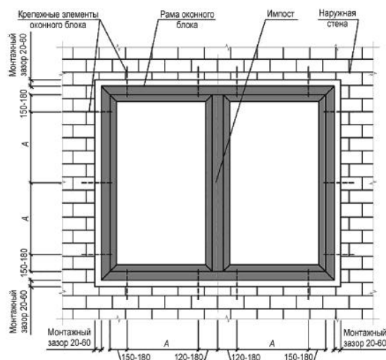
Рисунок 1 - Условия работы оконного блока
