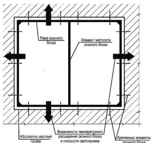
Рисунок 1 - Условия работы оконного блока
