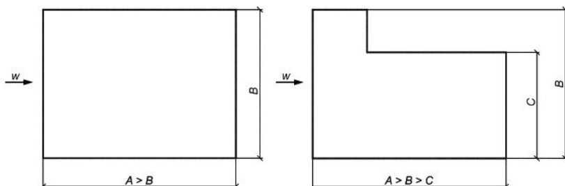
Рисунок Б.1 - Схема определения расчетного направления ветра
