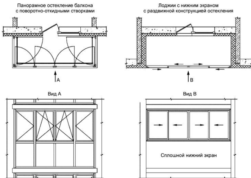
Рисунок Д.2 - Примеры конструкций наружного остекления
