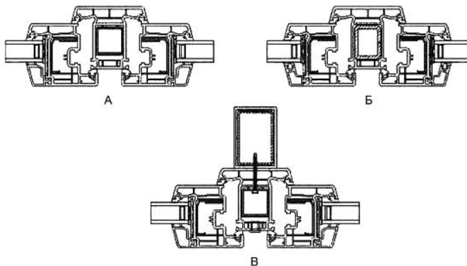
Рисунок Б.6 - Возможные конструктивные решения импоста оконного блока из поливинилхлоридных профилей
