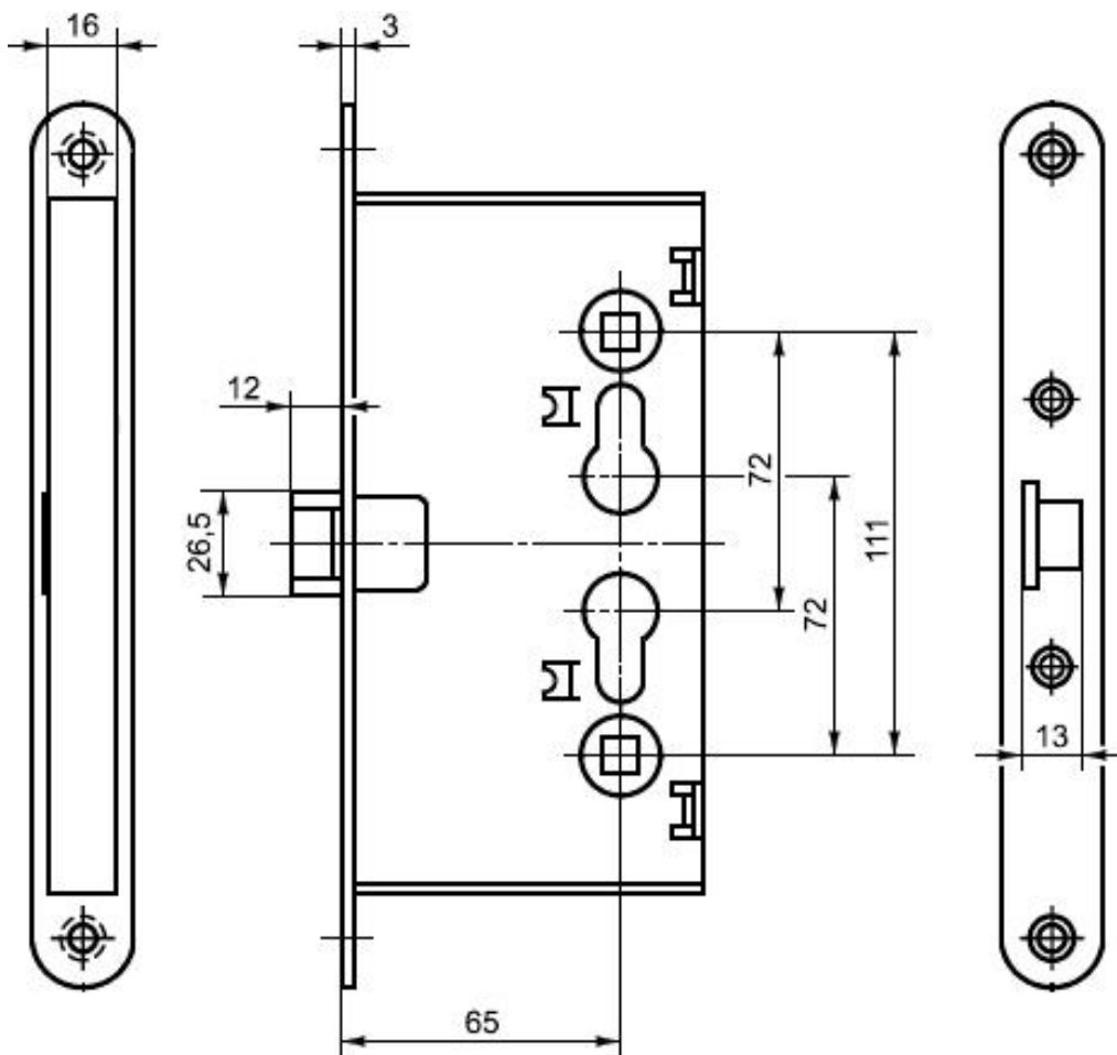
Рисунок Б.12 - Пример замка для противопожарной двери
