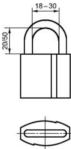
Рисунок Б.13 - Пример навесного замка типа ЗНВ1
