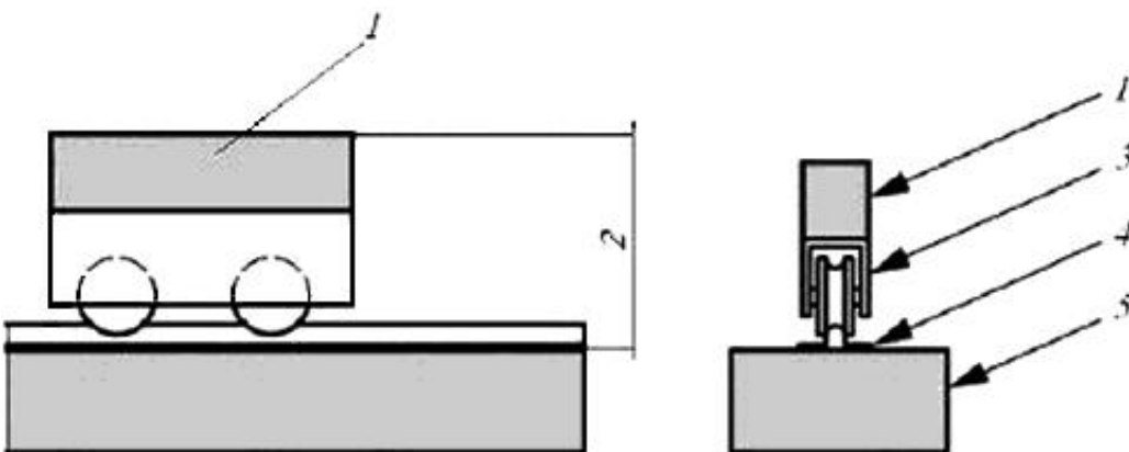
Рисунок Е.1 - Схема испытания роликов на надежность
