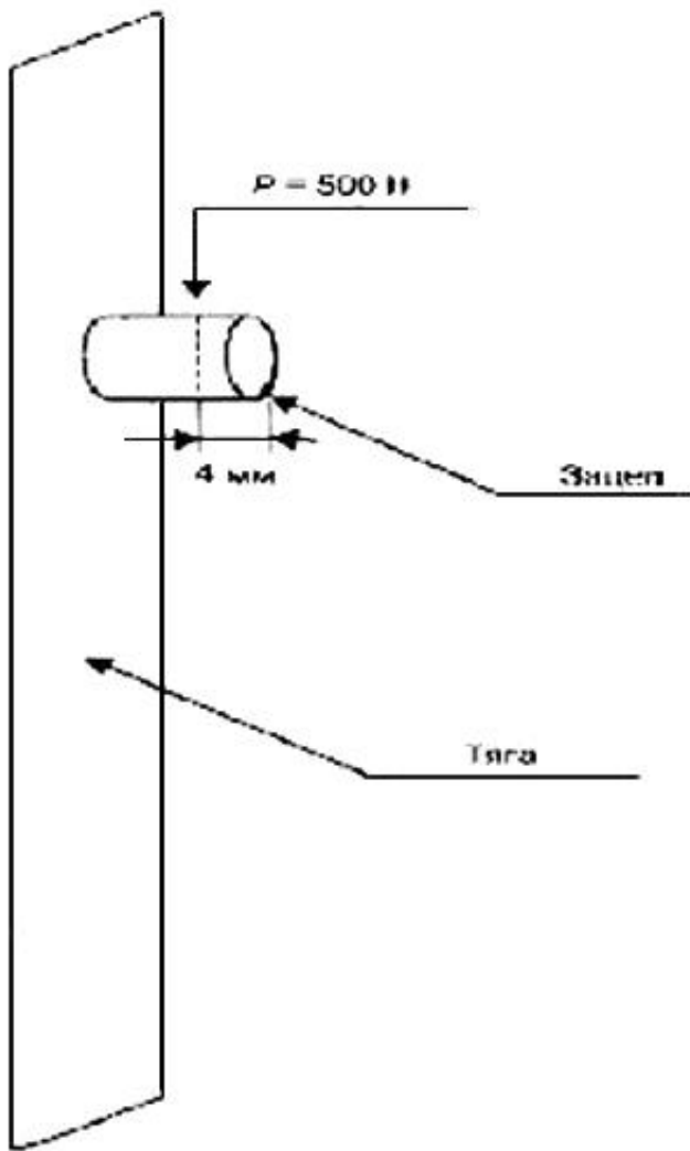
Рисунок Г.6 - Испытание крепления зацепа (см. 5.4.6)
