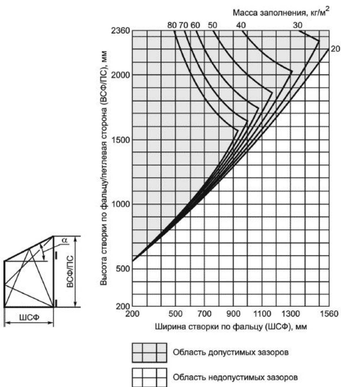
Рисунок В.4 - Диаграмма применения поворотно-откидных устройств для алюминиевых окон
