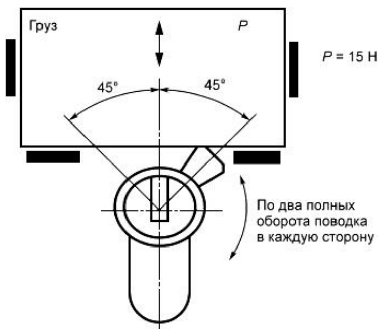
Рисунок 1 - Схема испытания цилиндрического механизма на наработку
