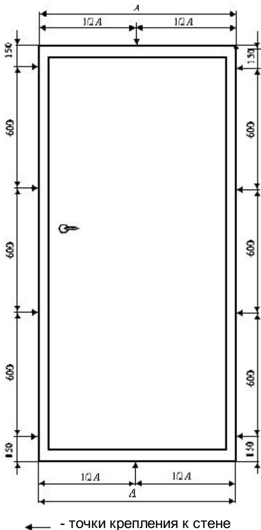
Рисунок А.2 - Пример расположения крепежных деталей при монтаже дверного блока с замкнутой коробкой
